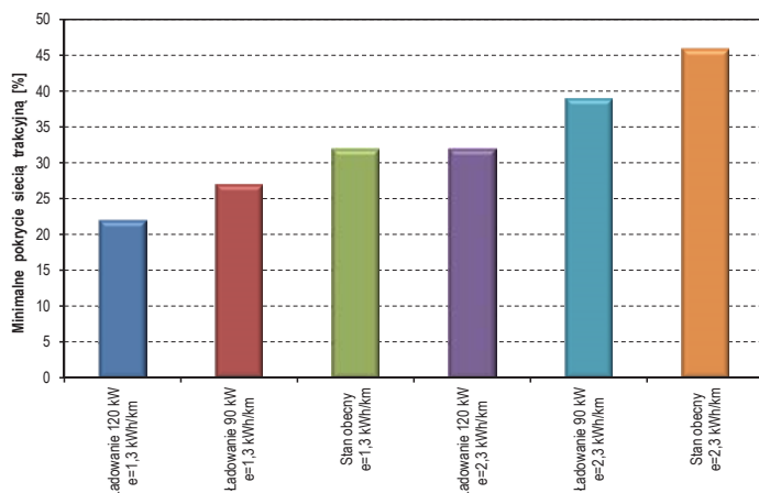
Rys. 5. Stopień minimalnego pokrycia sieci trakcyjną dla różnych warunków ruchu i ładowania
