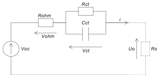
Rys. 6. Schemat zastępczy ogniwa litowo-jonowego [7]
